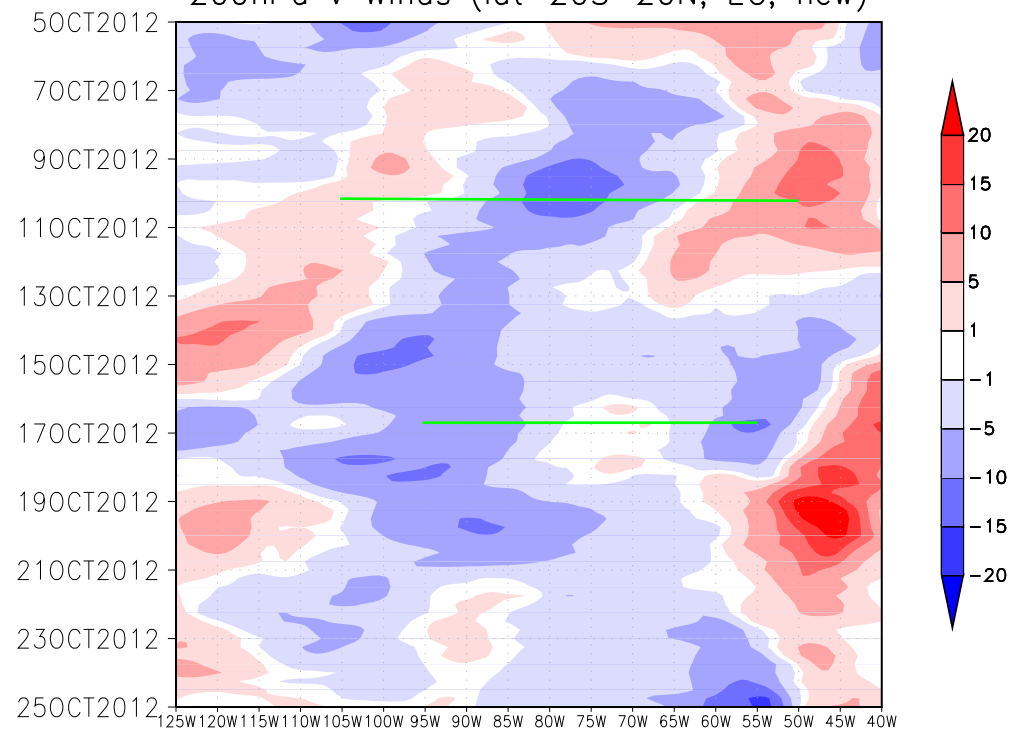
(d) 200hPa V Winds (lat=20S–20N, EC, new)
