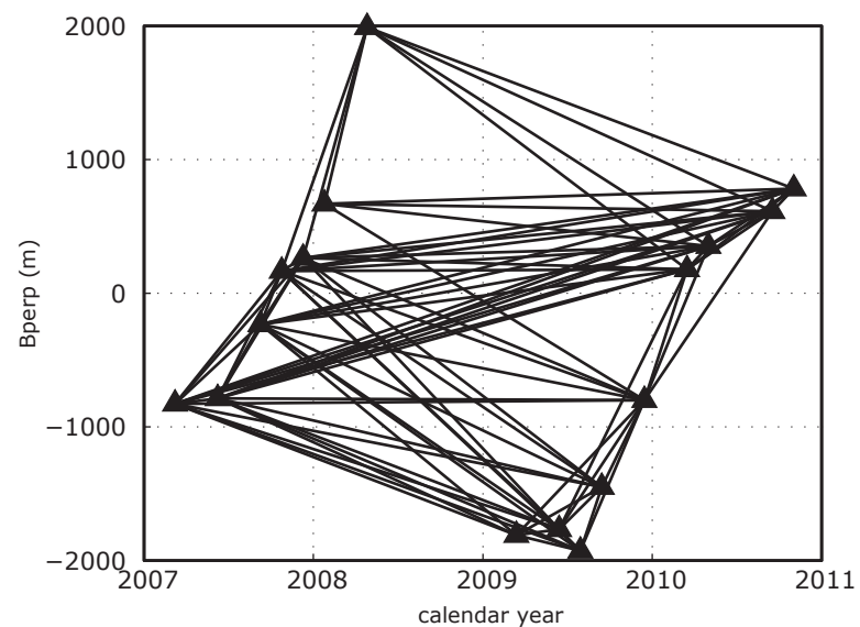
E) ENVISAT track 256, frame 2889, Nifg=34, Nsar=23
