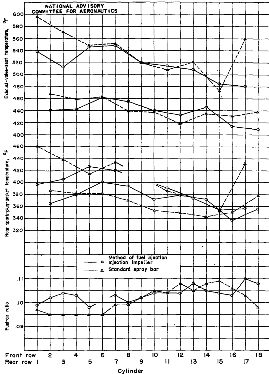
(d) Brake horsepower, 2000; engine speed, 2400 rpm.
